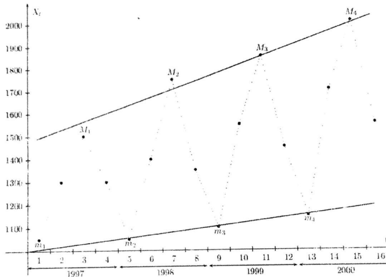
FIGURE 3.7 – Détermination du modèle - Méthode de la bande
