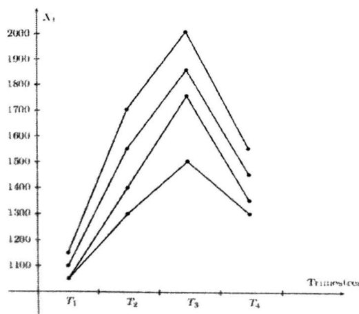
FIGURE 3.6 – Détermination du modèle - Méthode graphique de superposition
