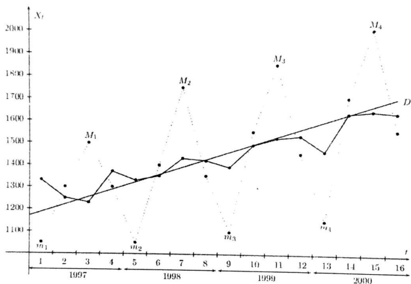
FIGURE 3.9 – Représentations graphiques de la série originale, de la droite de régression et de la série désaisonnalisée
