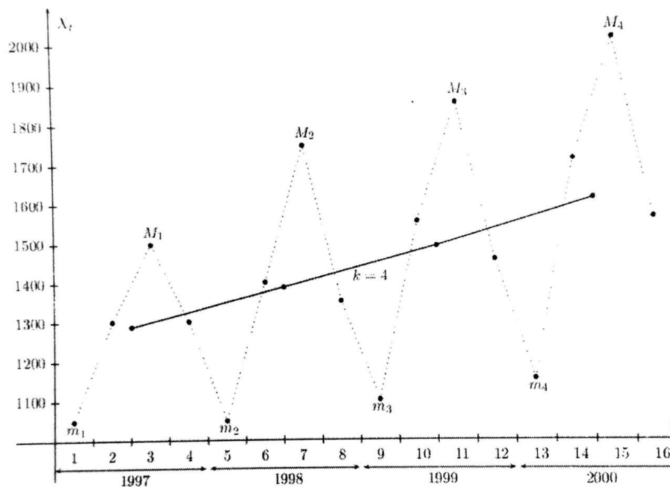
FIGURE 3.4 – Tendence - Moyennes échelonnées, k = 4
