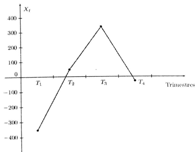
FIGURE 3.8 - Graphique des moyennes saisonnières
