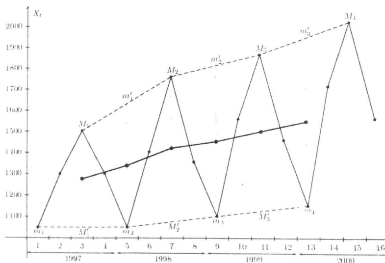
FIGURE 3.2 – Tendance - Méthode graphique
